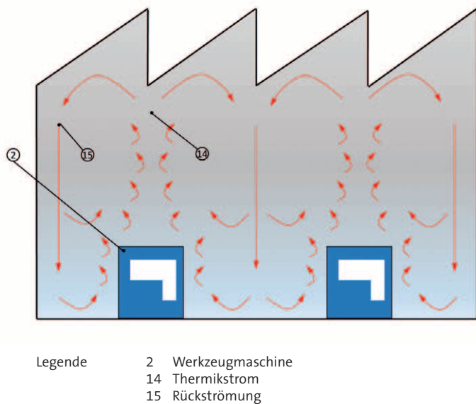
Bild 27 Thermikströme oberhalb warmer Oberflächen
