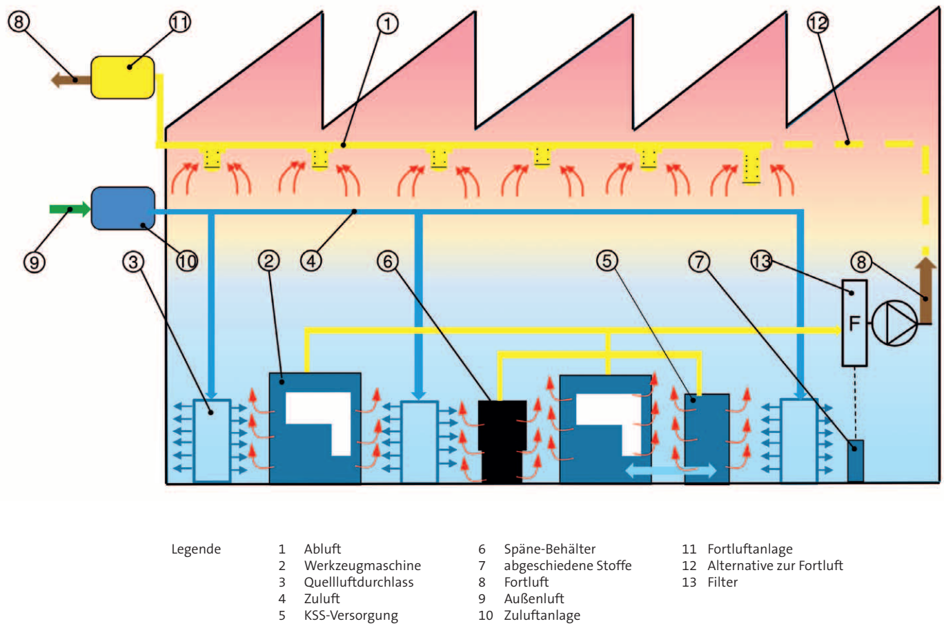
Bild 29 Beispiel eines optimalen Lüftungssystems
