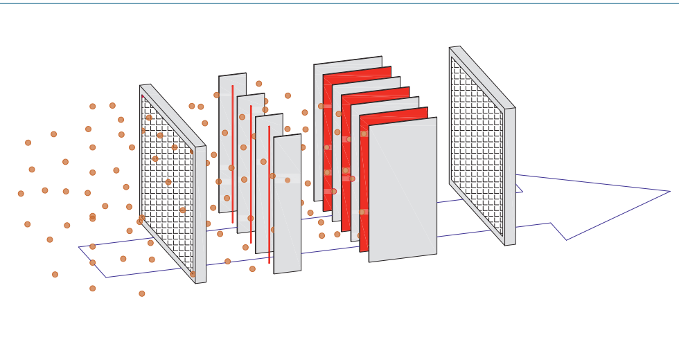
Bild 9 Funktionsprinzip Elektrofilter
