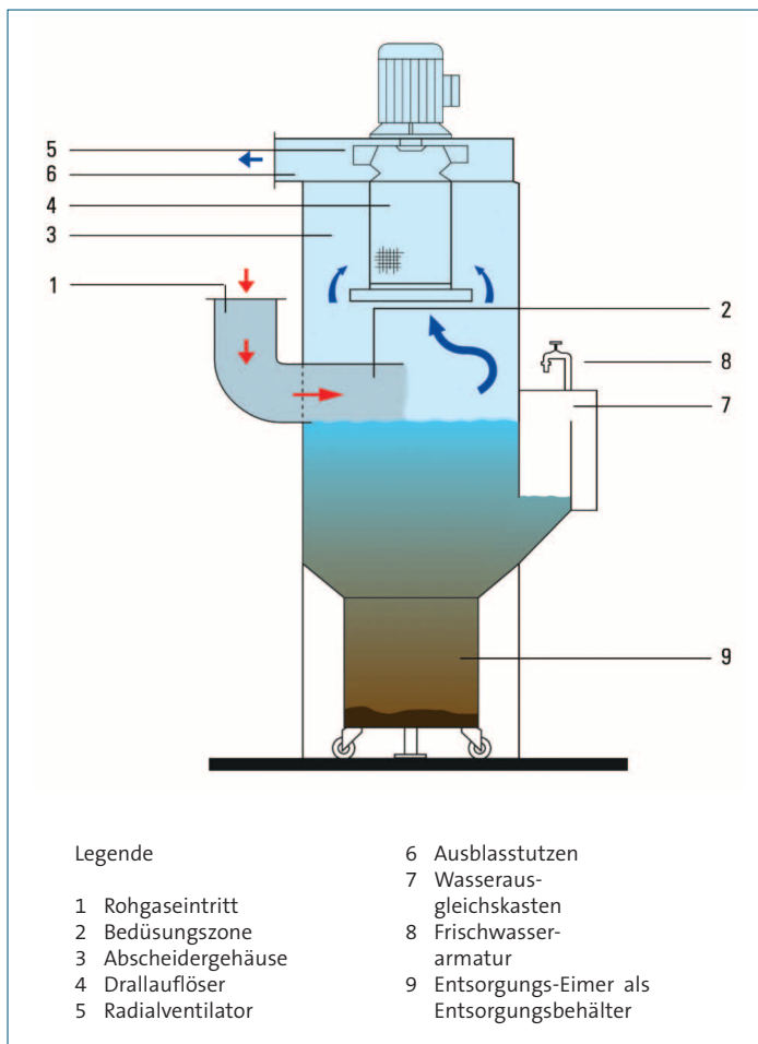
Bild 15 Funktionsprinzip Nassabscheider
