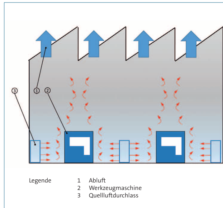
Bild 28 Schichtlüftung
