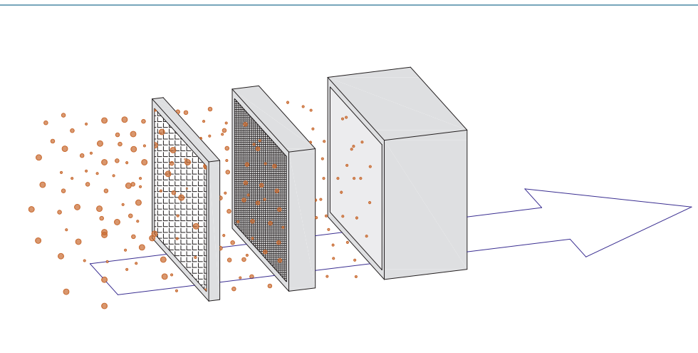
Bild 2 Filternde Abscheider
